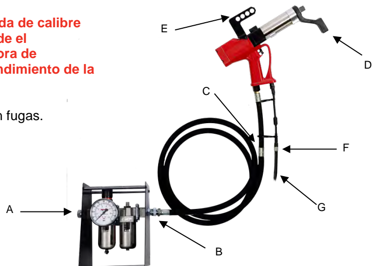
ILUSTRACIÓN 1 – Conexiones
