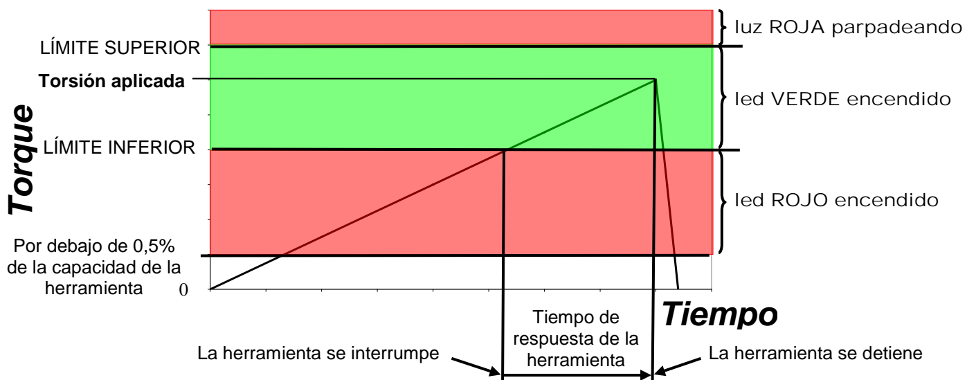
ILUSTRACIÓN 10 – Aplicación De Torsión Típica
