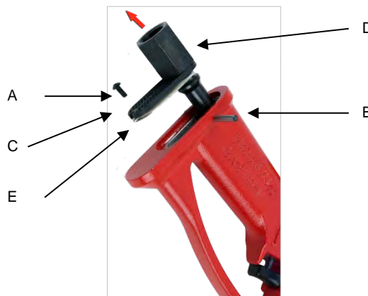
ILUSTRACIÓN 14 – Sustitución Del Silenciador
