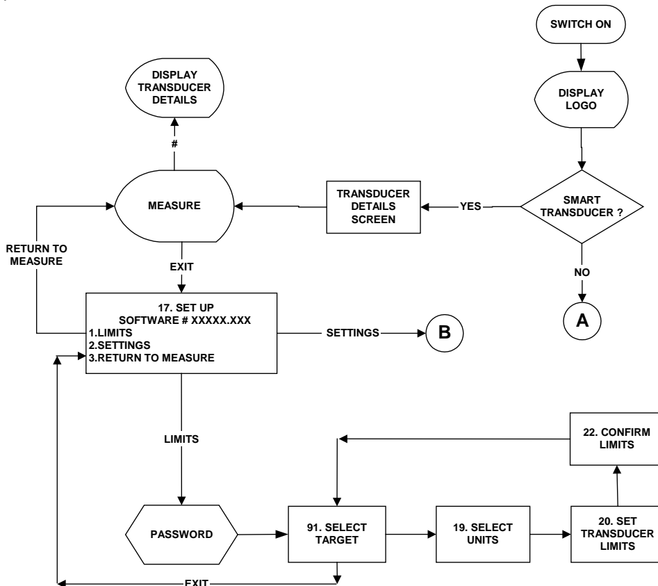
ILUSTRACIÓN 8 - Diagrama De Flujo Del Controlador De Herramientas
