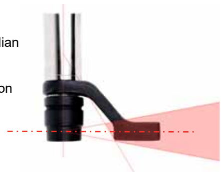
FIGURE 7 - Rayon de réactions sécuritaires pour douille de longueur
